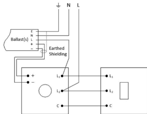
Maximum 1 dimmer per circuit
