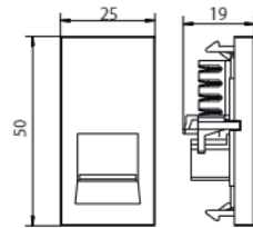
EMBTS1x
